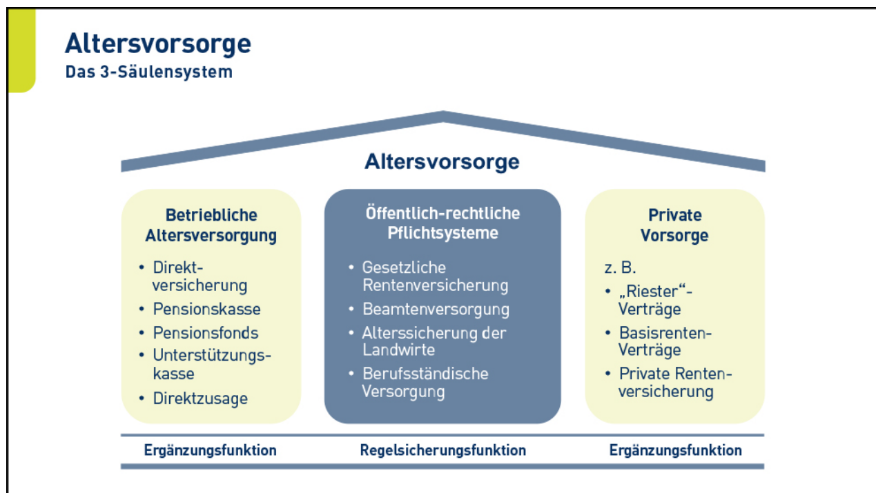
Abbildung 3: Das 3-Säulensystem
